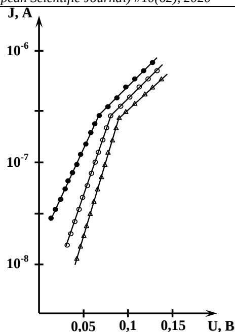
Рис.4. Рис. 4. Прямые ветви ВАХ от р-п структур на основе пленок PbTe легированной кислородом во время роста 77 К, 100 К, 120 К
