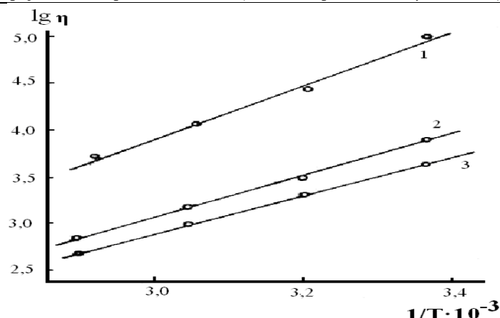
Рис.5. Зависимость \lg \eta от 1/T концентрированных растворов Na- KMЦ (1) и поликомплексных гелей Na-KMЦ –МФО с соотношением компонентов 4:1 (2) и 1:1 (3).
