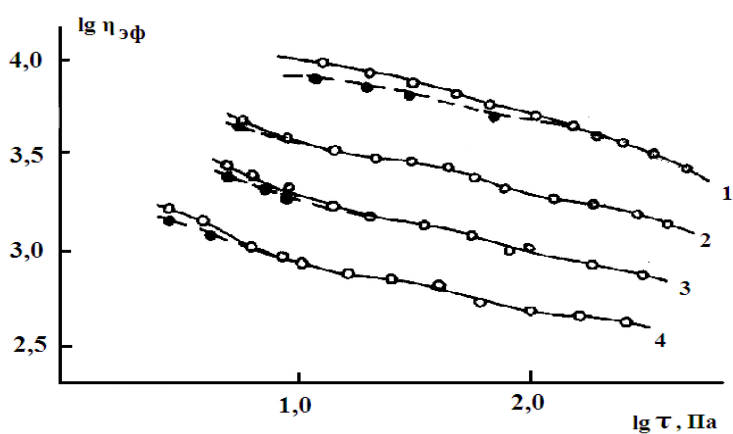
Рис.4. Кривые течения концентрированных систем ПКГ Na-КМЦ с МФО (4:1) при различной температуре T(K): 1 - 298, 2 - 313, 3 - 328, 4 - 343.
