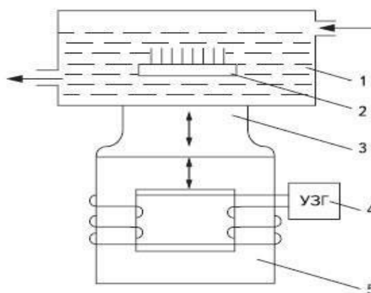
Рис. 2. Схема процесу ультразвукового очищення в протоці розчинника 1 - ванна; 2 - касета з пластинами; 3 - концентратор; 4 - Генератор ультразвукових коливань; 5 - магнітострикційний випромінювач
