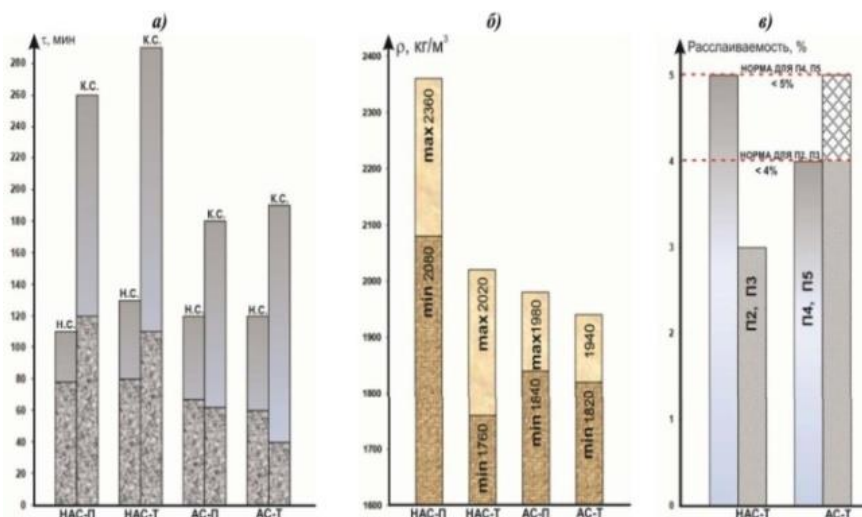
Рис. 2. Изменение абсолютных значений свойств растворных смесей: а) – сроков схватывания; б) – плотности; раслаиваемости – НАС/П и НАС/Т – 1 и 2 неактивированные; АС/П и АС/Т – 3 и 4 активированные
