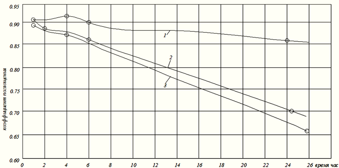
Рис.4. Изменение коэффициента поглощения бетона солнечной спектра с Ж = 20-25 сек;
