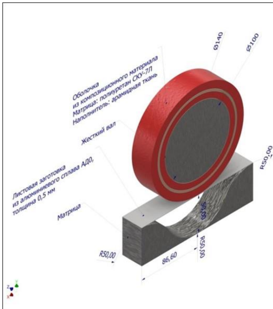
Рисунок 3 – Схема нагружения
