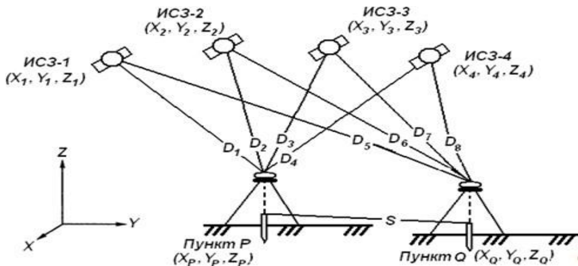
Рис. 2 - Относительный метод определения координат
