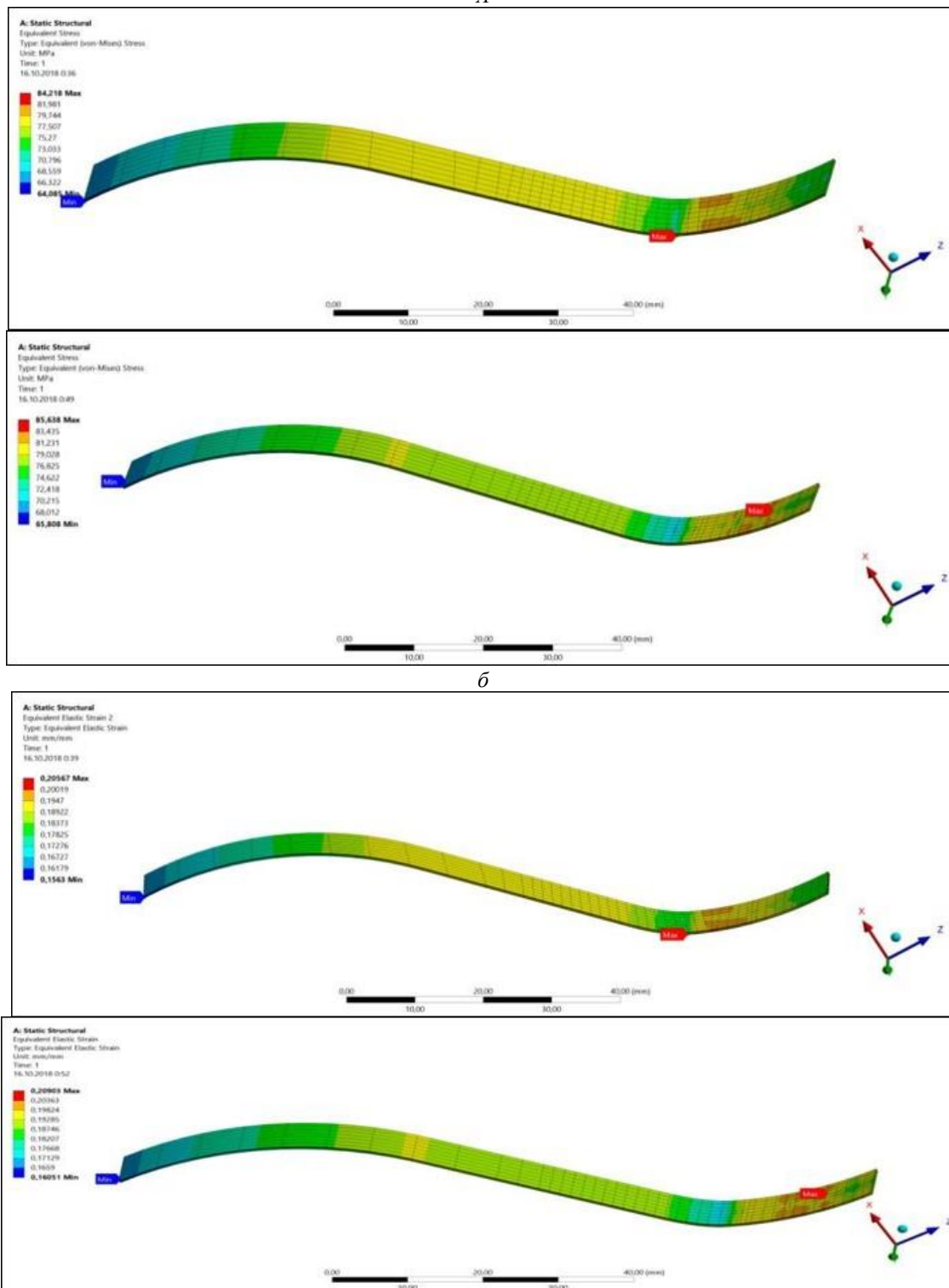
Рисунок 5 (а,б)- а - эквивалентные напряжения, б – эквивалентные деформации
