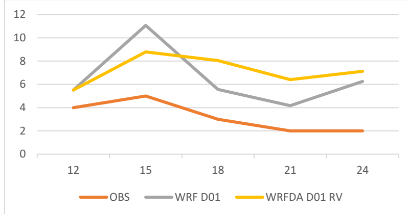
Рис. 8. График распределения скорости ветра на 10 м (м/с) на станции Столбцы, OBS – наблюдения, WRF D01 – без ассимиляции, WRFDA D01 RV – с ассимиляцией, 18.02.2020 г.
