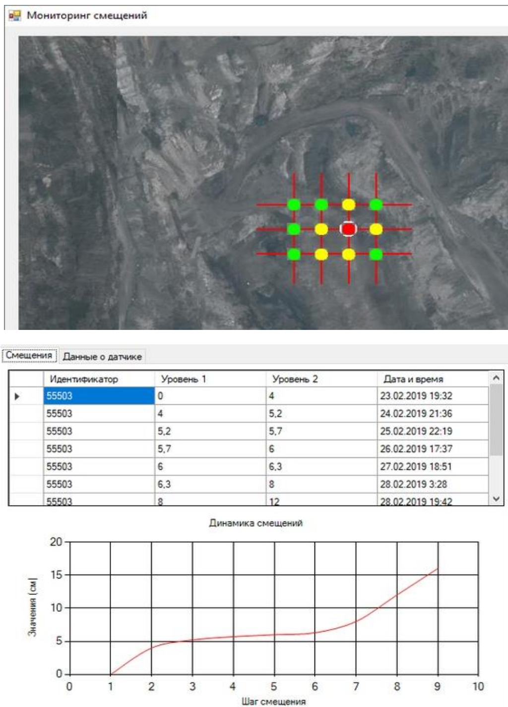
Рис. 2. Интерфейс программы
