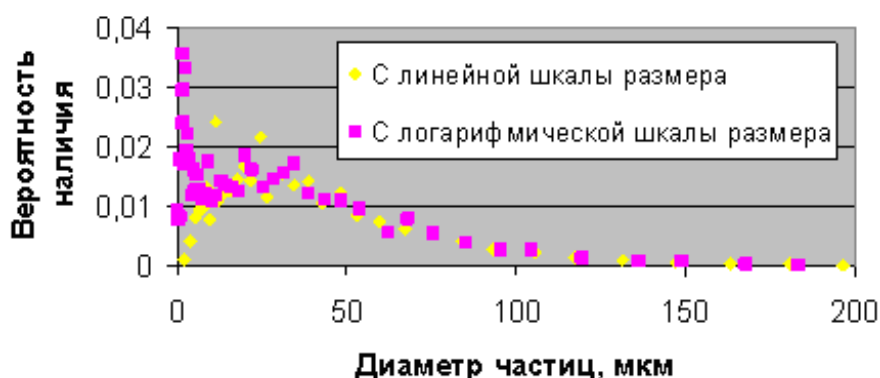
Рис. 6. Сопоставление результатов оцифровки данных дисперсионного анализа металлообразивной пыли: сравниваются данные, полученные на основе линейной (желтые точки) и логарифмической (розовые точки) размерных шкал
