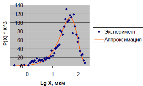
Рис. 9. Аппроксимация экспериментальных данных распределением Розина – Рамллера P(x) = 7.73 \cdot 10^{-3} \cdot 0.322 \cdot \exp[-(x/48.89)1.322] (левый фрагмент, среднеквадратичная относительная погрешность составляет 0.47, коэффициент корреляции с экспериментальными точками 0.972) и трехпараметрическим распределением P(x) = 6.66 \cdot 10^{-3} \cdot 0.4 \cdot \exp[-(x/66.18)1.235] (правый фрагмент, среднеквадратичная относительная погрешность составляет 0.51, коэффициент корреляции с экспериментальными точками 0.972)
