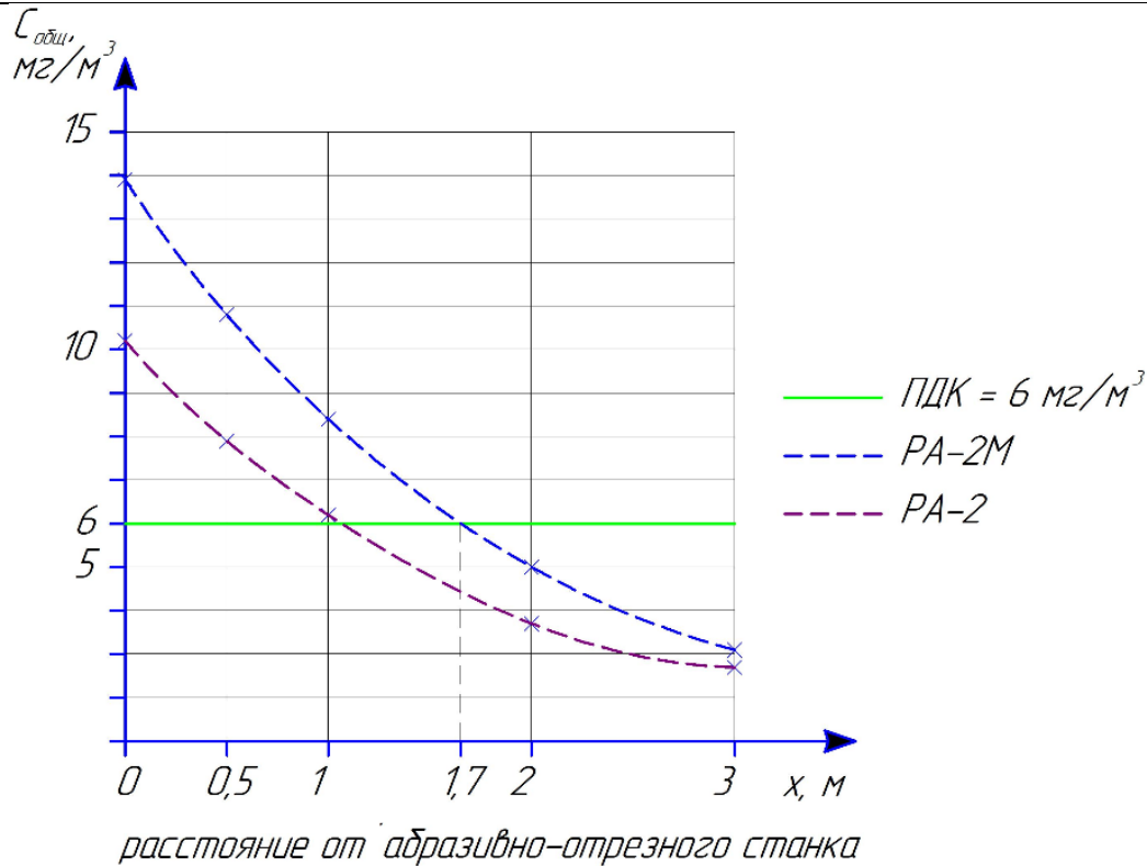
Рис. 4. Запыленность в зоне дыхания работника и на удалении от рельсорезного станка при отсутствии пыле- и шумозащитного кожуха
