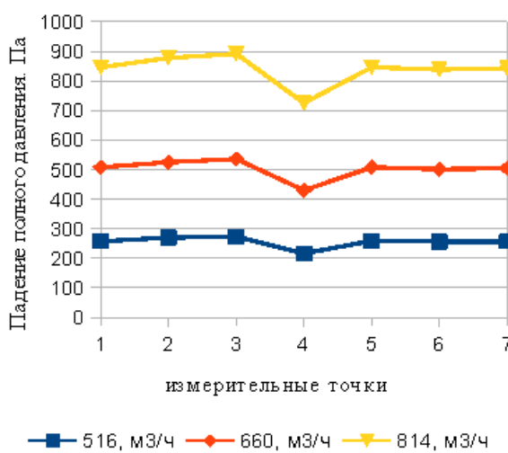
Рис. 12. Потери давления для циклонов «ЦН15у-300» (слева) и «ЦОК-200-300» (справа) при различной производительности вентилятора
