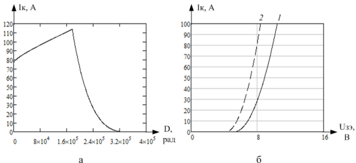
Рис. 5. Зависимость тока коллектора от поглощенной дозы (а) и передаточные характеристики БТИЗ (б): 1 – до облучения, 2 – после облучения
