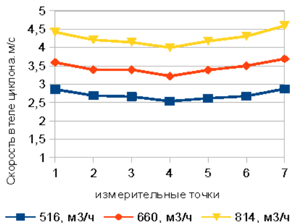
Рис. 11. Скорость потока в теле циклонов «ЦН15у-300» (слева) и «ЦОК-200-300» (справа) при различной производительности вентилятора
