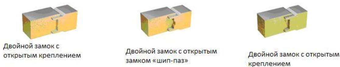
Рисунок 1 - Общий вид вариантов крепления типа «шип-паз» сэндвич-панелей
