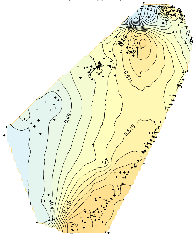
Рис.1.12. Вероятностная схема перспектив нефтегазоносности по показателям P(vr-ir) , P(vr-ar_1) и P(vr-ar_2) для территории ПС
