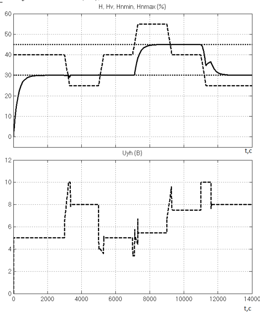
Рис. 4. Графики изменения переменных канала регулирования влажности: H_v(t) , H(t) , H_{min}(t) , H_{max}(t) , U_{yh}(t)
