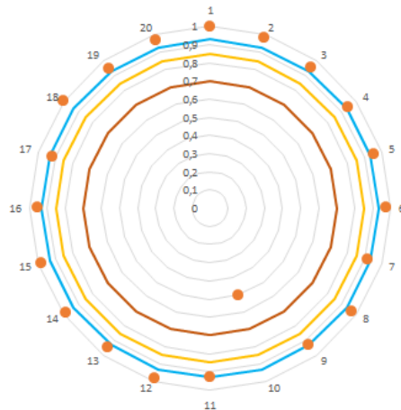
Рис. 2. Корреляция частных экспертных мнений с коллективным средним. Номер эксперта на круговой диаграмме увеличивается по часовой стрелке; большая окружность соответствует уровню корреляции 0,93, средняя – 0,85, малая – 0,7
