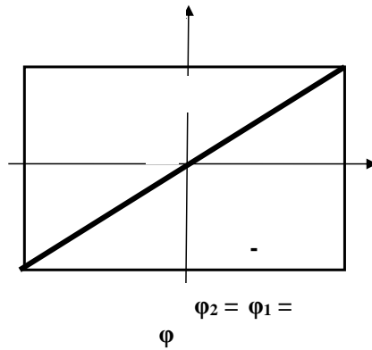
Рис. 5. Векторное представление траектория движения частицы [10 -11]
