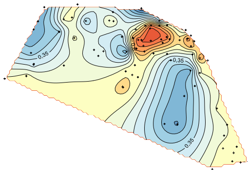
Рис.1.9. Вероятностная схема перспектив нефтегазоносности по показателю P_{\text{КОМ}}^{\text{СП}} для зоны НГТР 3-А
