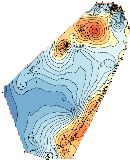
Рис.1.13. Вероятностная схема перспектив нефтегазоносности по показателю R_{КОМ}^{СП} для территории ПК
