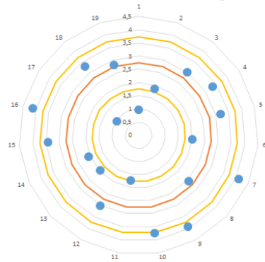
Рис. 5. Отклонение частных экспертных мнений от коллективного среднего
